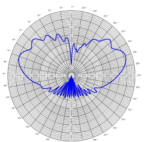
ROLL 4.75 GHz
