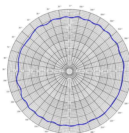
AZIMUTH (YAW) 4.75 GHz
